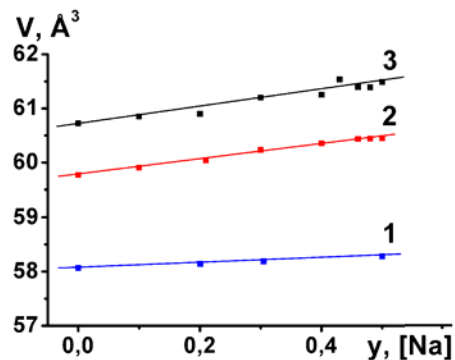
Рис. 1. Залежності об'єму елементарної комірки від концентрації натрію ( y ) в системах \text{Li}_{0.5-y}\text{Na}_y\text{La}_{0.5}\text{TiO}_3 (1) [9], \text{Li}_{0.5-y}\text{Na}_y\text{La}_{0.5}\bullet\text{Nb}_2\text{O}_6 (2) та \text{Li}_{0.5-y}\text{Na}_y\text{La}_{0.5}\bullet\text{Ta}_2\text{O}_6 (3).
